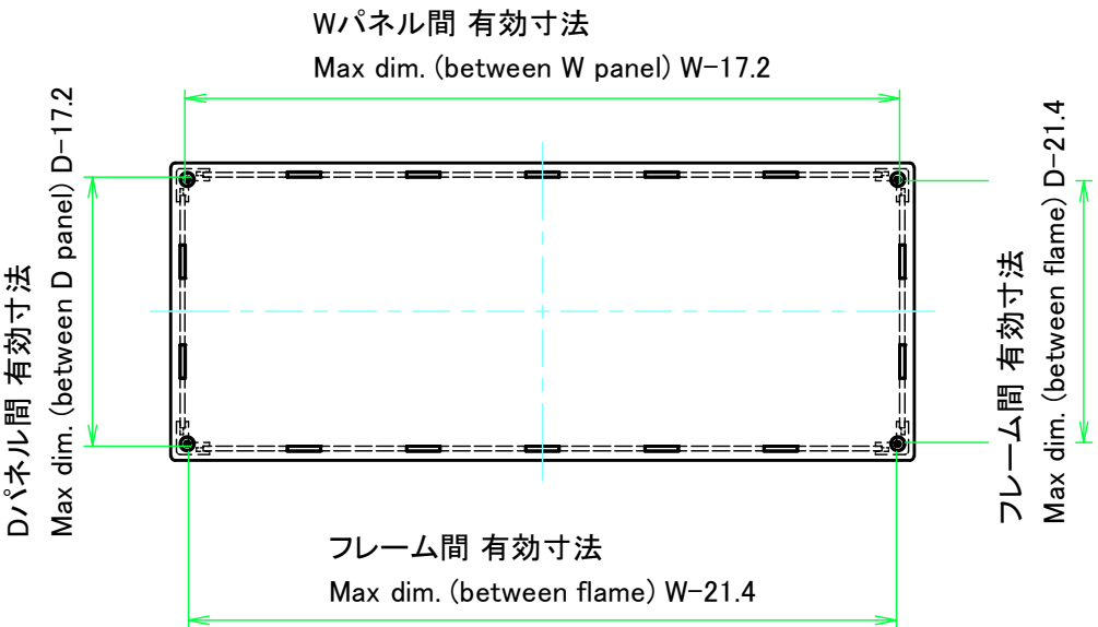
下カバー / Bottom cover
